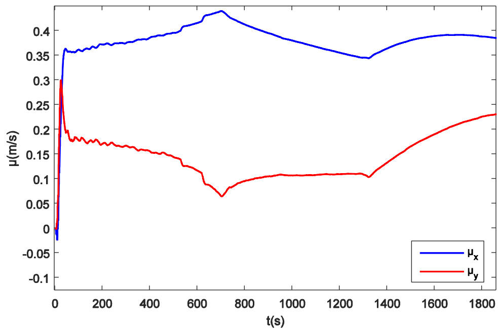
Figura 5 Velocidad de las corrientes estimada.
