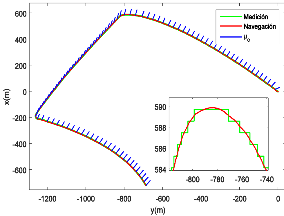
Figura 4 Trayectoria descrita por el vehículo.
