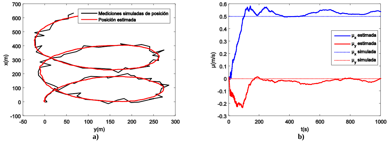
Figura 2 Trayectoria descrita por el vehículo.
