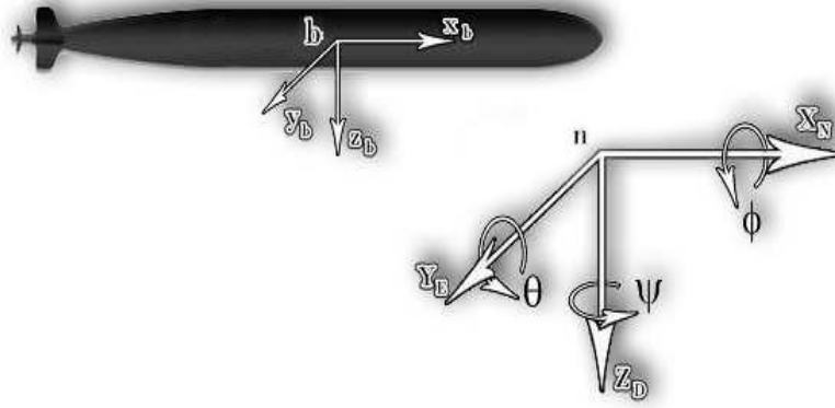
Figura 1 Sistemas de referencia.
