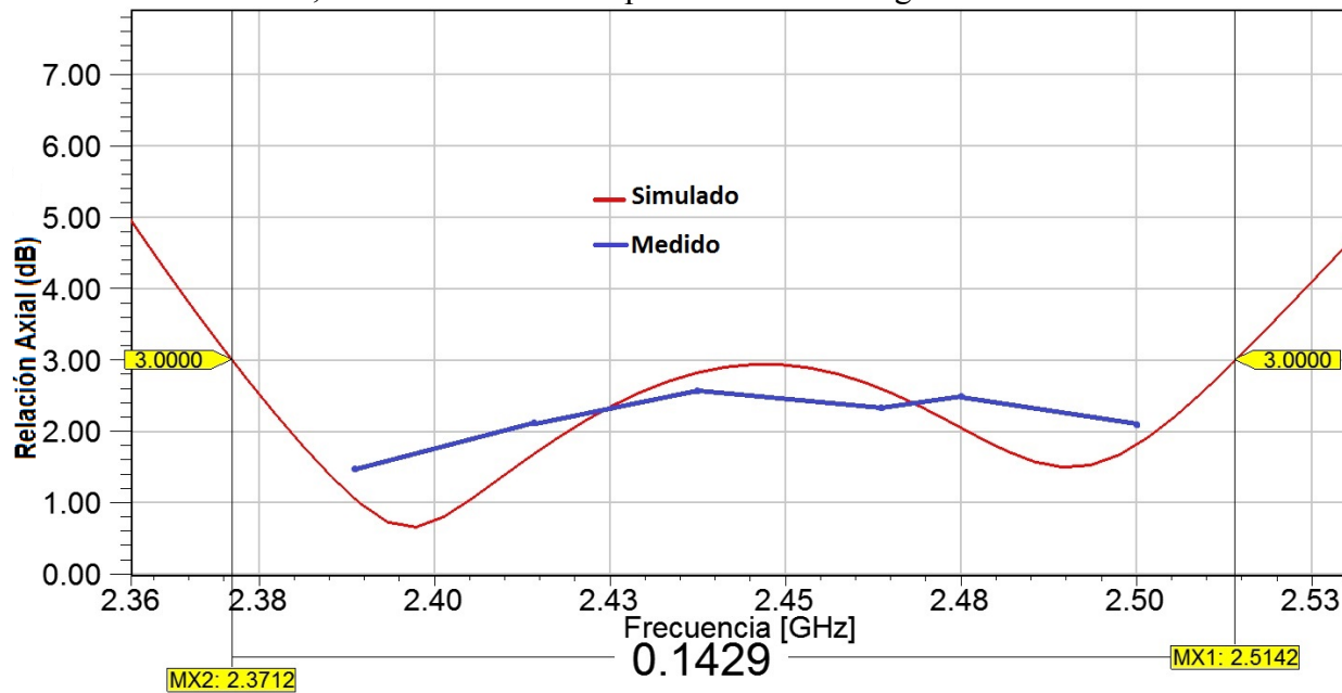
Figura 14 Relación axial simulada y medida.
