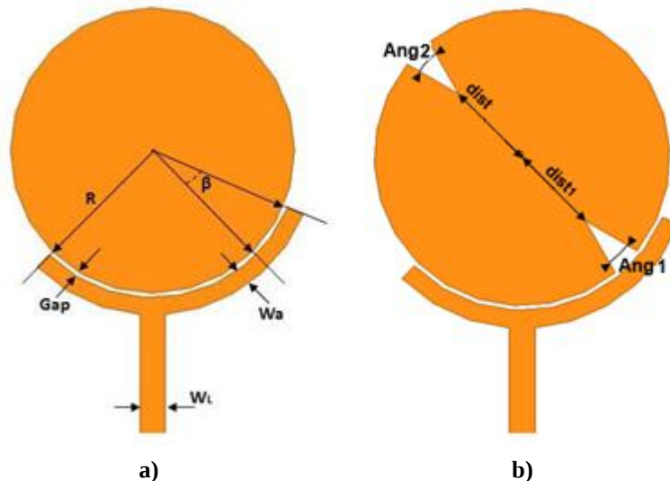
Figura 2 a) Diseño con desfasaje en la alimentación. b) Diseño con ranuras en los bordes.
