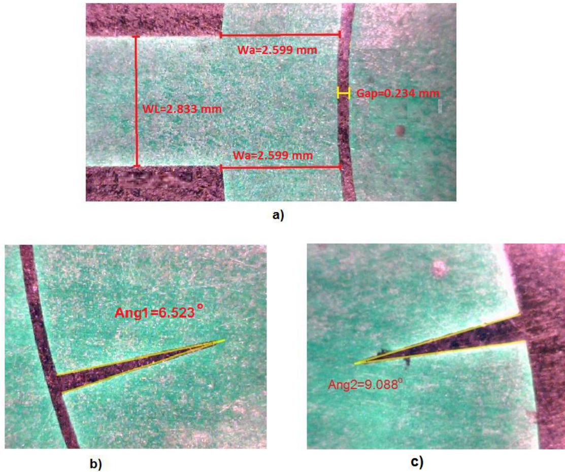
Figura 9 Dimensiones de la antena construida a) Alimentación b) Ang1 c) Ang2.
